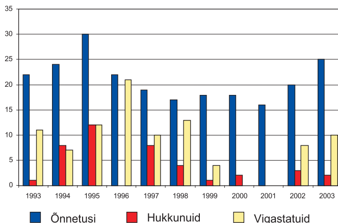
Joonis 2. Liiklusõnnetuste arvu, hukkunute ja vigastatute arvu dünaamika 1993–2003 raudteeülesõidukohtadel
