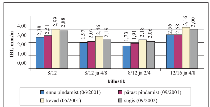
Joonis 3. Keskmise IRI Tallinn–Tartu maantee katselõikudel
