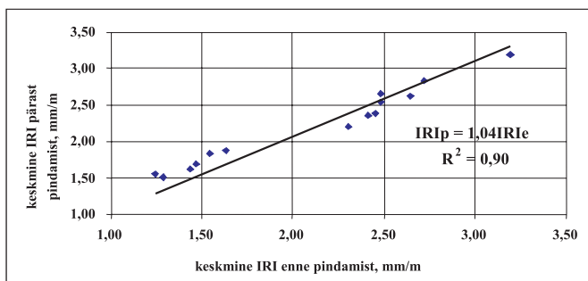
Joonis 1. IRI enne ja pärast pindamist
