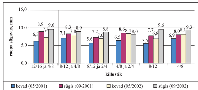
Joonis 8. Keskmise roopa sügavus Ääsmäe–Rohuküla maantee katselõikudel
