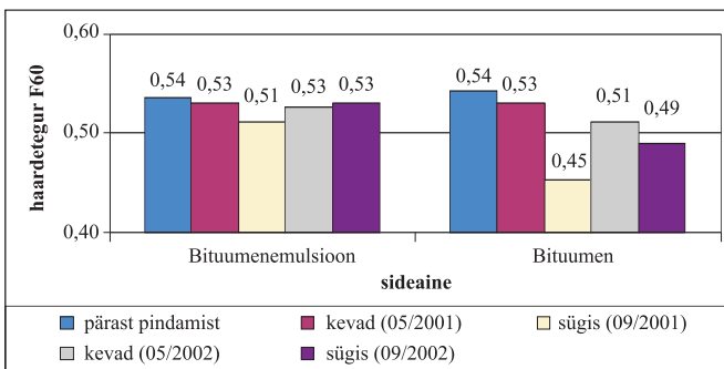
Joonis 11. Keskmine haardetegur F60 Ääsmäe-Rohuküla maantee katselõikudel
