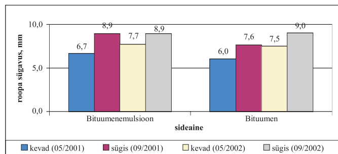
Joonis 9. Keskmise roopa sügavus Ääsmäe–Rohuküla maantee katselõikudel
